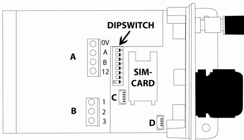
Fig 1. Kretskortets ovansida
