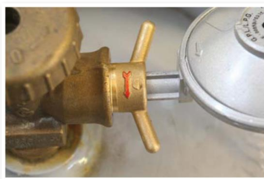
Vasenkierteinen liitos
