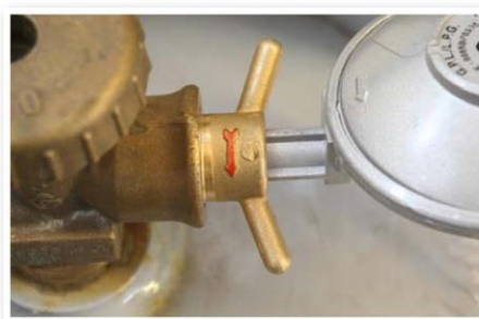
Vänstergängad anslutning
