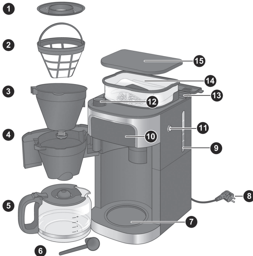
Fig. 1: Apparats dele
