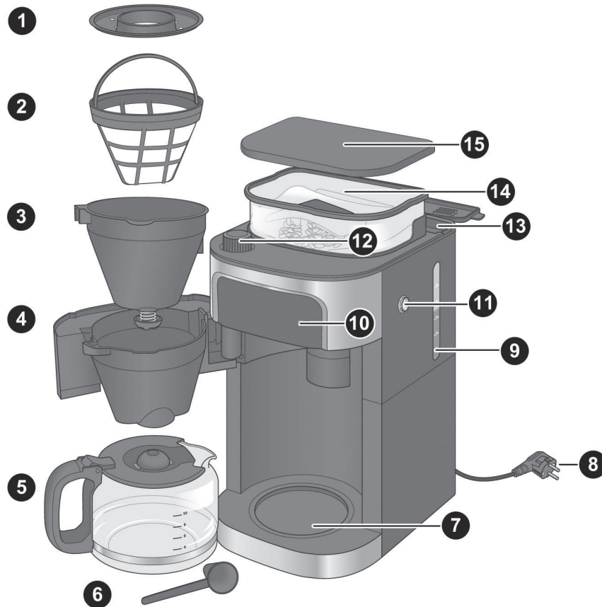
Fig. 1: Parti dell'apparecchio
