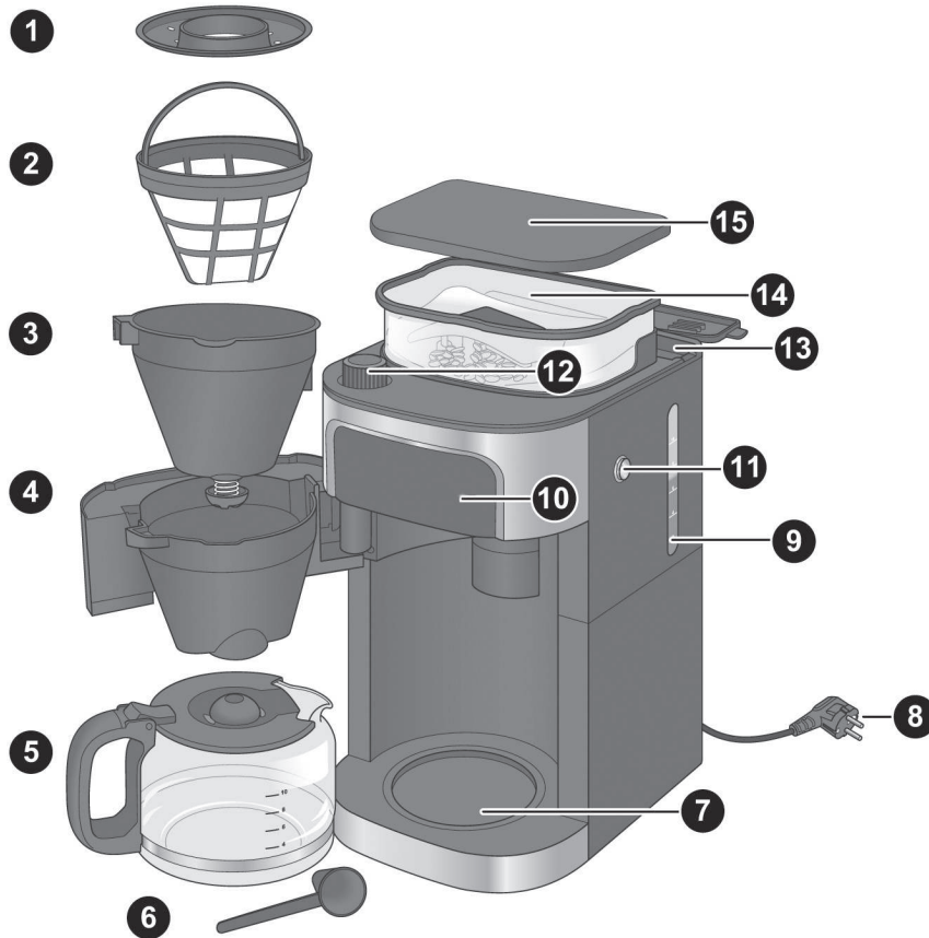
Bild 1: Apparats delar
