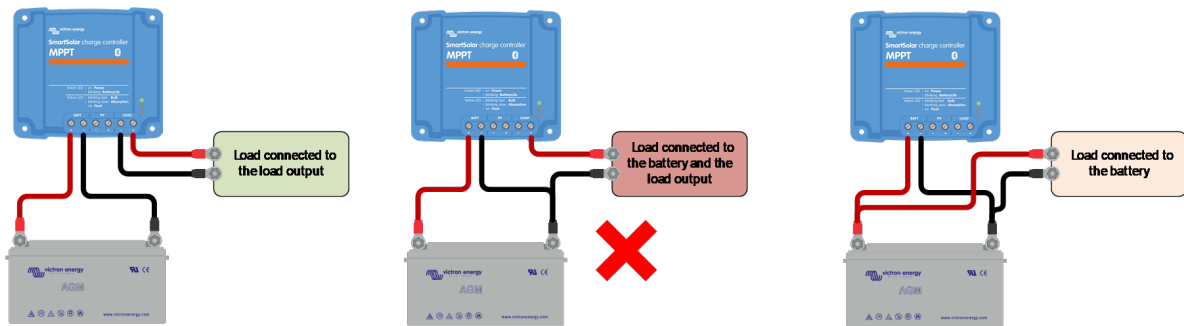
Fullständig belastningsströmvälsläsning
